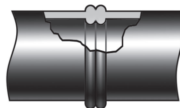
Рис. 4.2.1. Соединение труб сваркой встык
