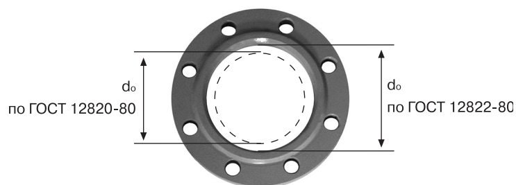
Рис. 1.2. Фланец свободный металлический по ГОСТ 12822-80 (рис. 1.2) отличается от фланца приварного по ГОСТ 12820-80 только увеличенным внутренним диаметром d_1 , что позволяет свободно надеть его на ПЭ трубу
