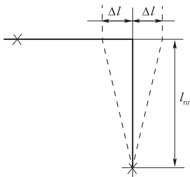
Рис. 2.4. Г-образный поворот
