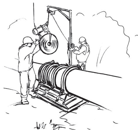
Рис. 4.2.7. Введение торцевателя для механической обработки торцов свариваемых поверхностей труб
